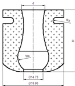
钨钢喷嘴
