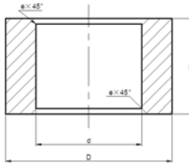
钨钢塞规-LS型
